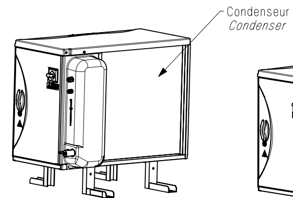
MONTAGE AU SOL FLOOR MOUNTING
